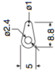
Solder Lug
